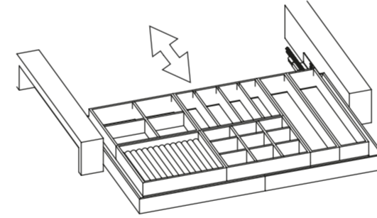
Raylı Mücevherlik Jewel Rail
